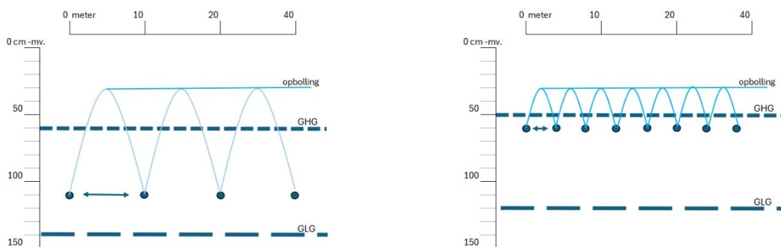
Figuur 3: schematische weergave van reguliere drainage (links) en hoger en nauwer draineren (rechts). Met de blauwe stippen is de drainagebasis aangegeven. De GHG is niet hetzelfde als de maximale opbolling, omdat de GHG een gemiddelde grondwaterstand is en de opbolling afhankelijk is van de beschikbaarheid van water (regen, verdamping).
