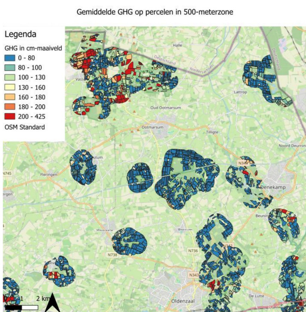
Figuur 1. Gemiddeld hoogste grondwaterstand per perceel in een aantal van de 500-meterzones rondom natuurgebieden. Bron: KK-kaart Vechtstromen
