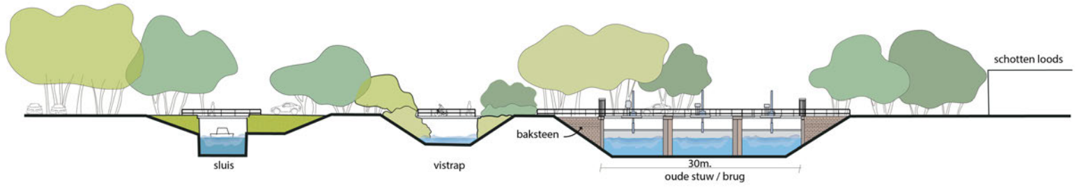
Doorsnede-aanzicht stuw Junne in nieuwe situatie
