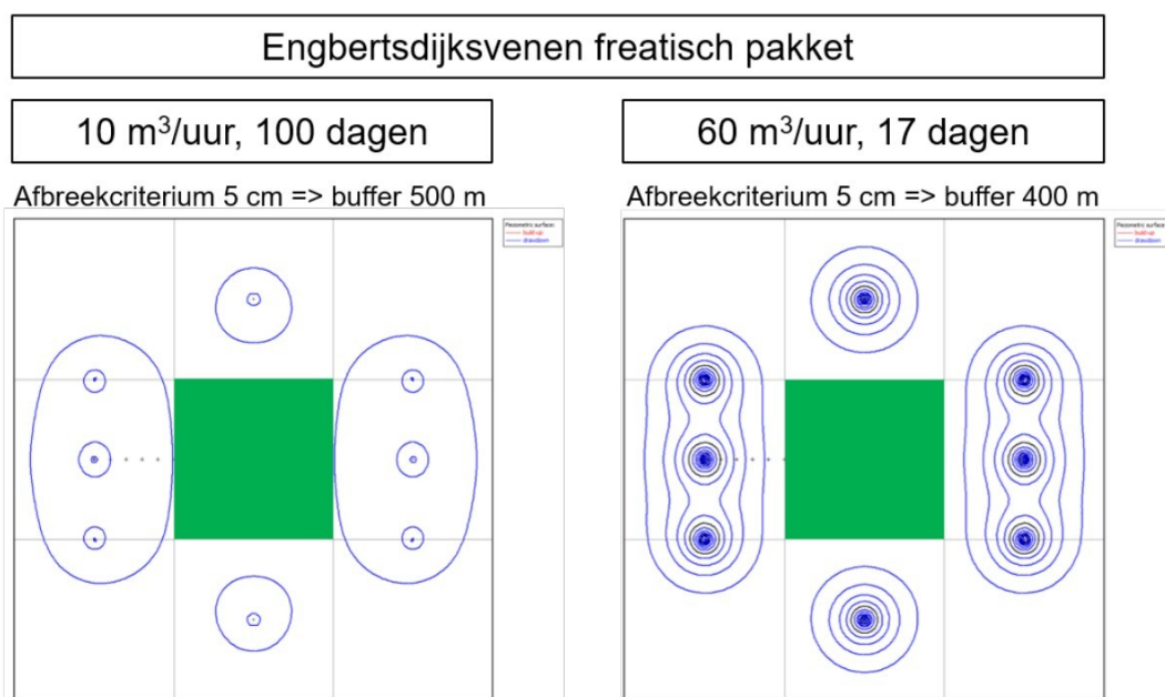
Figuur 3-6 Berekende verlagingcontouren bij onttrekking rondom geschematiseerd natuurgebied van 1 * 1 km op basis van bodemschematisatie EDV, netwerk in bovenstaande figuren is 1 * 1 km, buitenste verlagingcontour is 0,05 m.
