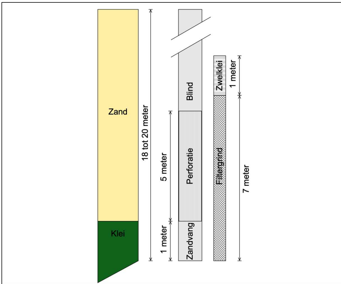
Figuur 14 – Opstelling bron
