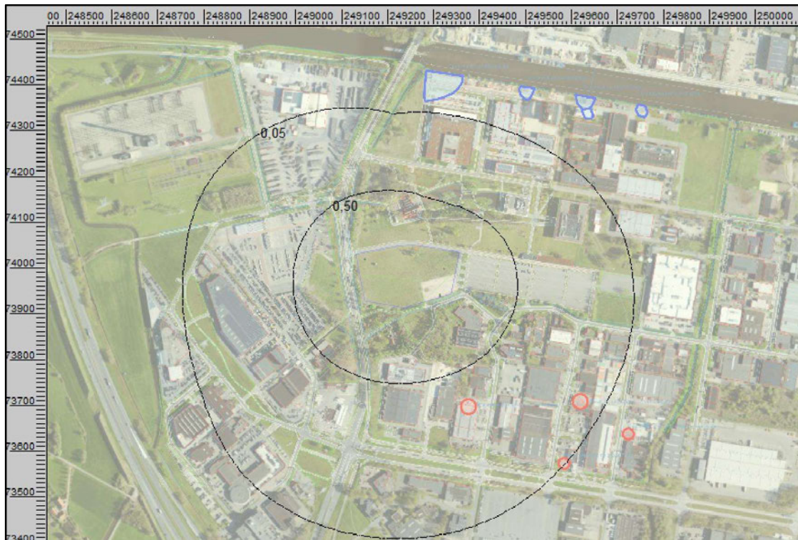
Figuur 21 - Grondwaterverontreinigingen
