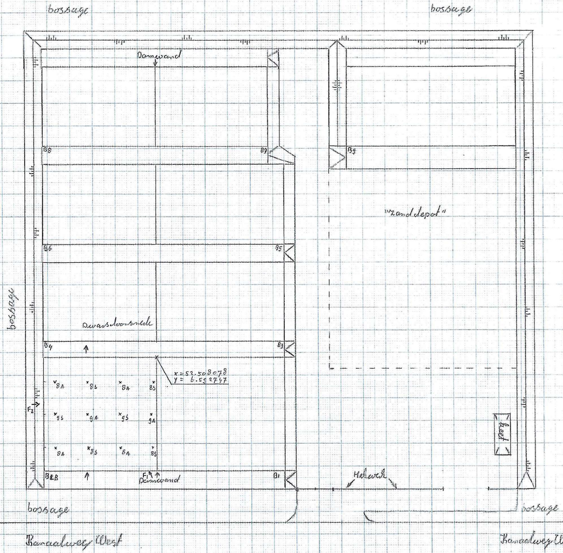
Dwarsdoorsnede 1:200
